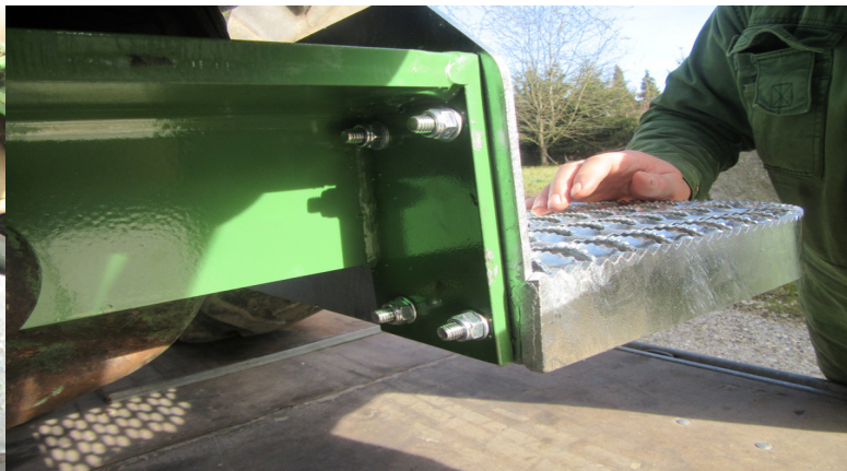
Auftritt mit 4 Schrauben 8x25 u. Beilagscheiben 8,4x16 am Tritthalter anschrauben
