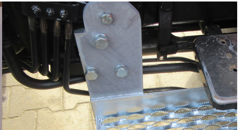
Halter wird mit 4 Schrauben mit Sprengring am Ge- triebeblock verschraubt
