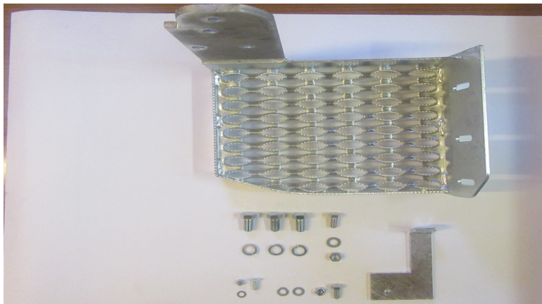
Lieferumfang: Auftritt mit Halterung, Gegenhalter und Schraubensatz
