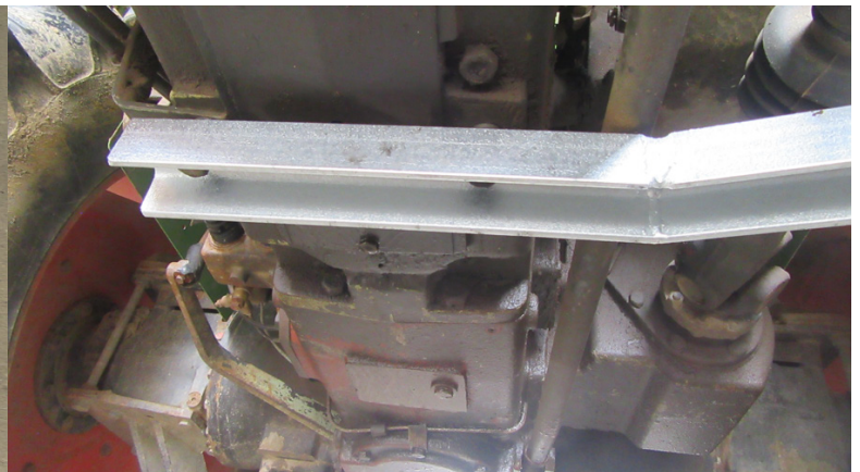
Tritthalter wird mit 2 Schrauben 12x50 mit Spreng-ring am Getriebeblock befestigt
