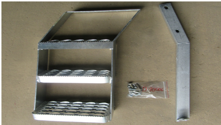
Lieferumfang: Tritthalter, Trittleiter 3-sprossig, Schraubensatz
